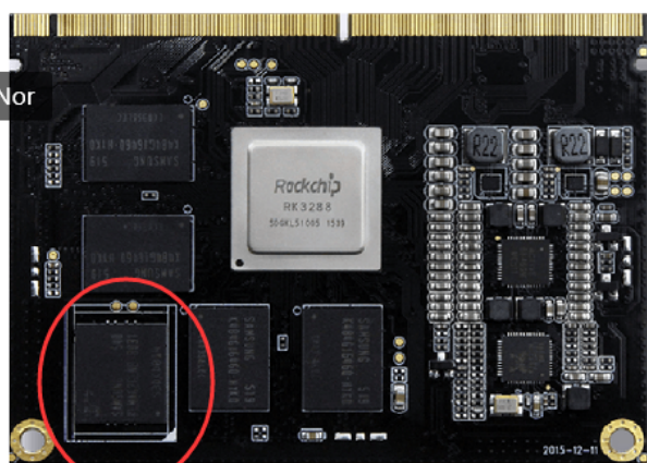
1 EMMC
