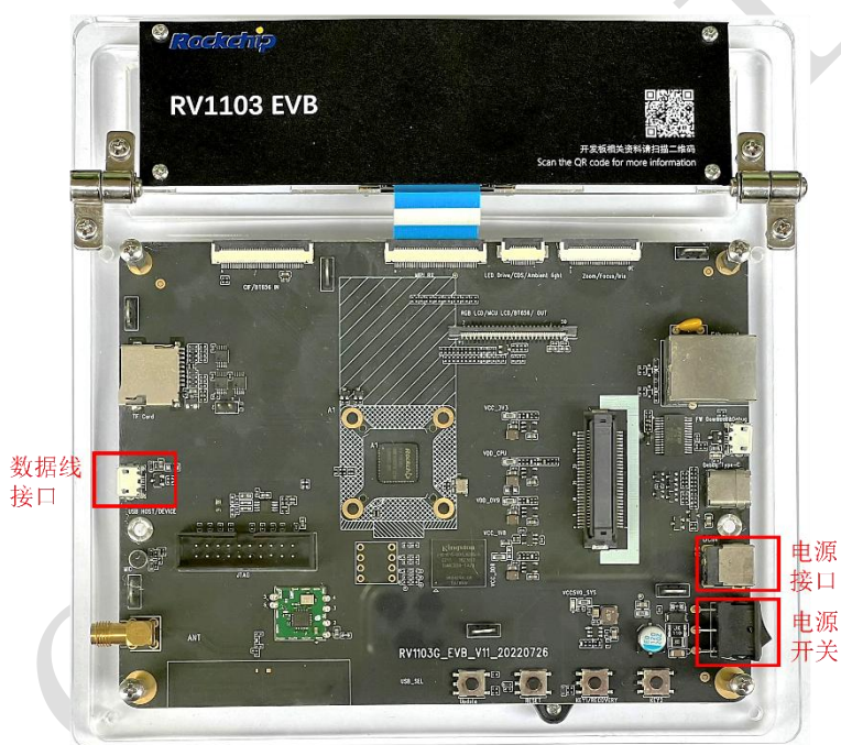
图 2-1 RV1103 开发板
