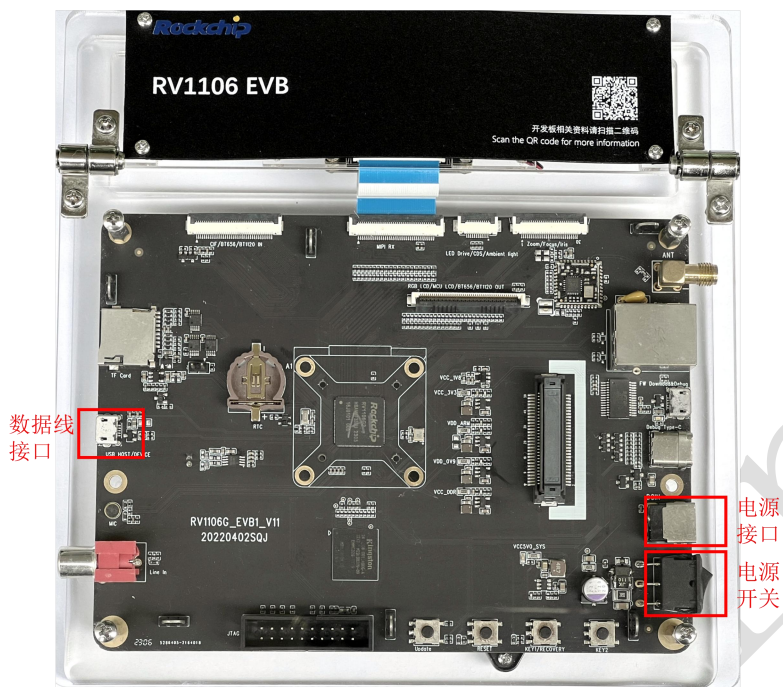
图 2-5 RV1106 开发板
